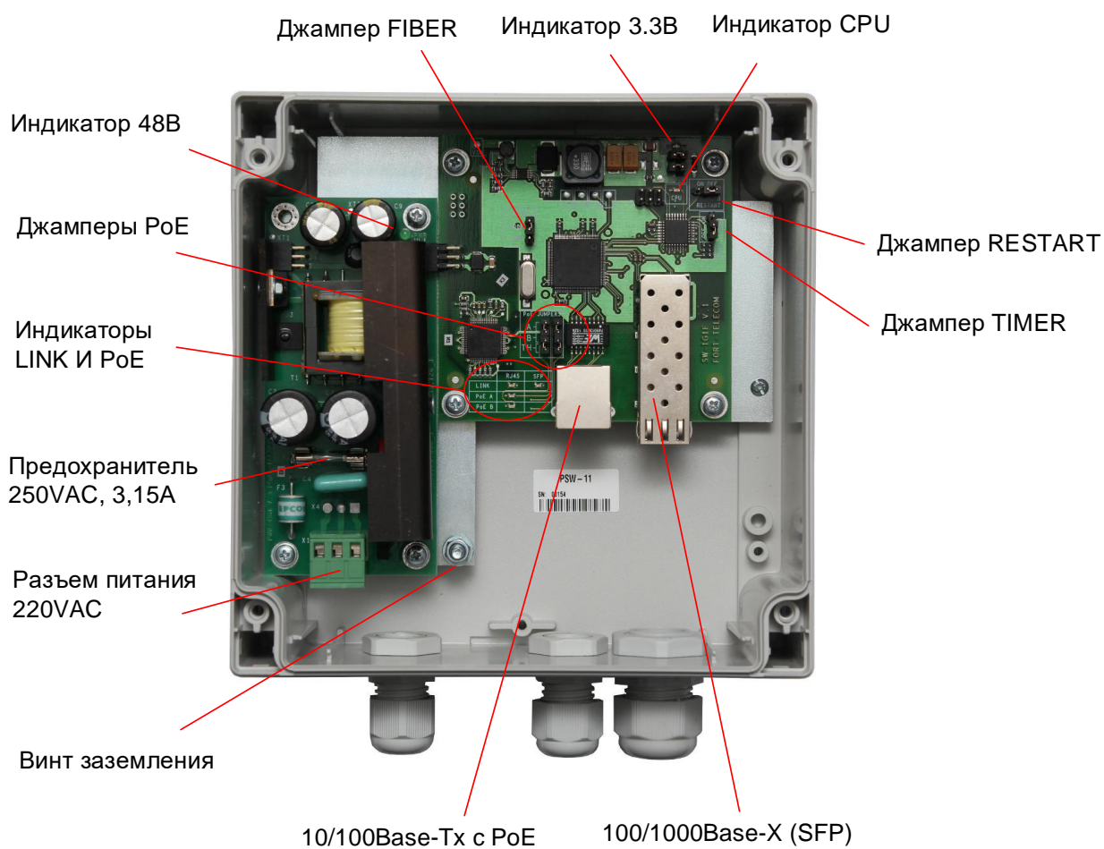
Рисунок 2.2.1 - Расположение элементов PSW -11
