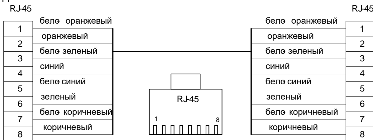
Рисунок 6.4 - Разделка кабеля.
